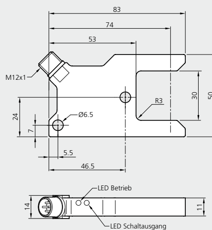
Stahlgehäuse verzinkt Steel casing galvanized
