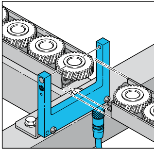
Teileerfassung in Zuführschienen (OGU ...) Part detection in supply guides (OGU ...)
